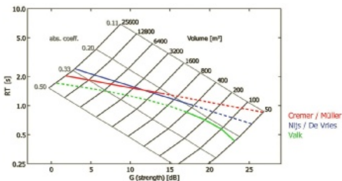
Figuur 3: Vergelijking verschillende modellen voor beschrijving van gewenste akoestiek in een G-RT-diagram.
