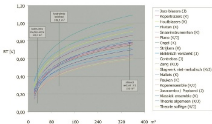
Figuur 4: De gewenste akoestiek, uitgedrukt in de nagalmtijd, voor verschillende instrumentgroepen.
