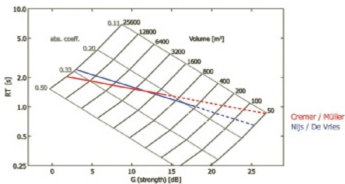
Figuur 1: Beschrijving gewenste nagalmtijd voor zalen door Cremer en Müller en Nijs en de Vries in een G - RT -diagram. De horizontale as geeft de luidheid, aangeduid met de Engelse term G (strength).
